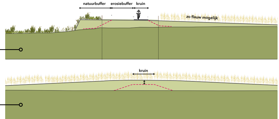
Figuur 5 - Twee innovatieve dijkconcepten in Limburg, de steilranddijk (boven) en de hoge grond (beneden).
